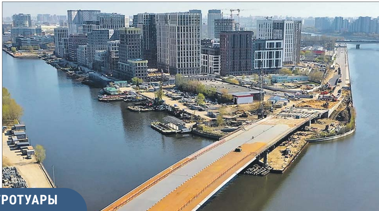
Центральный пролёт установили на постоянные опоры
